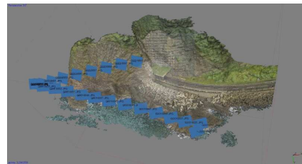
写真-UAV 画像より 3D 地形を作成
